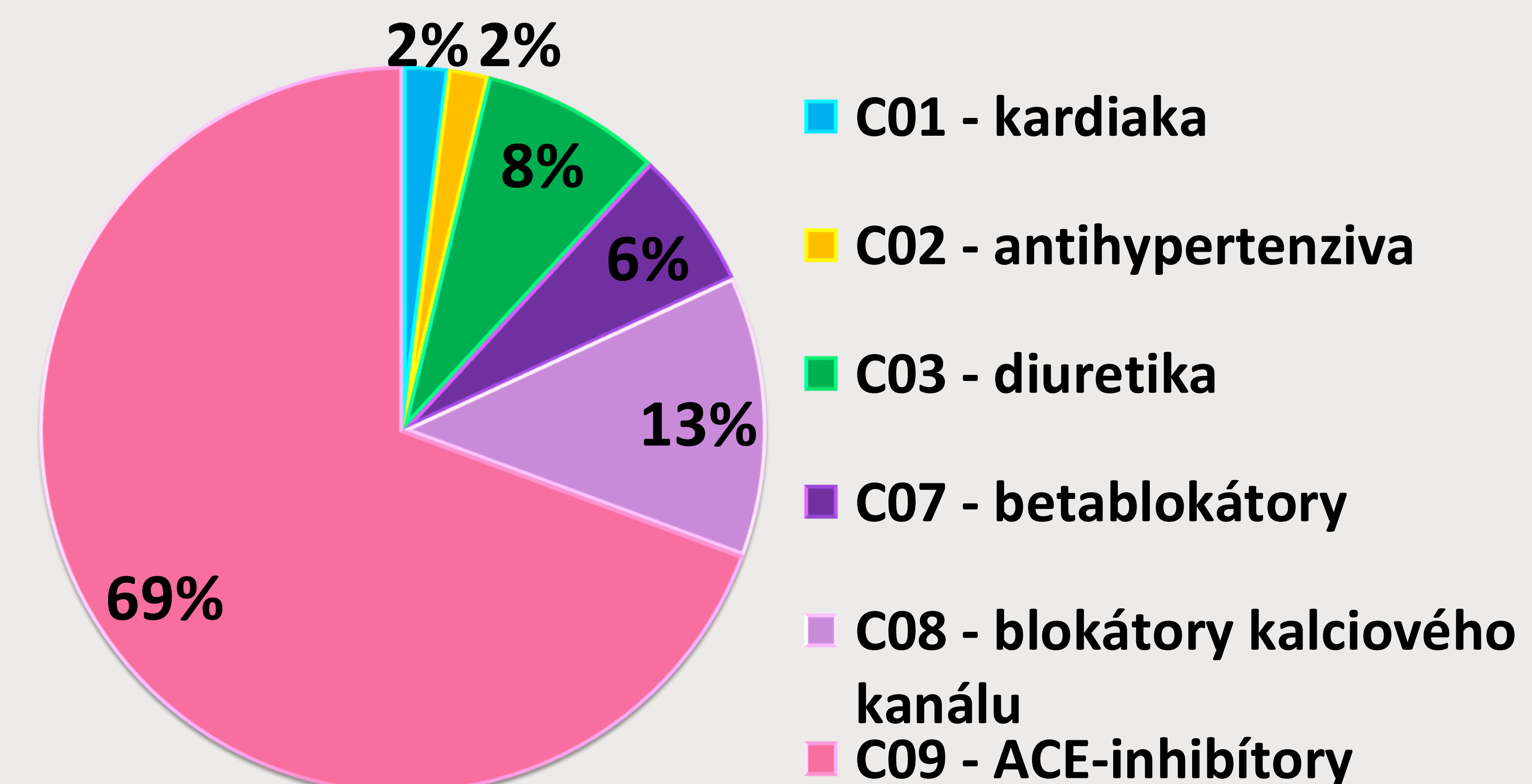
Graf č. 2 – Četnost preskripce dle ATC skupin
