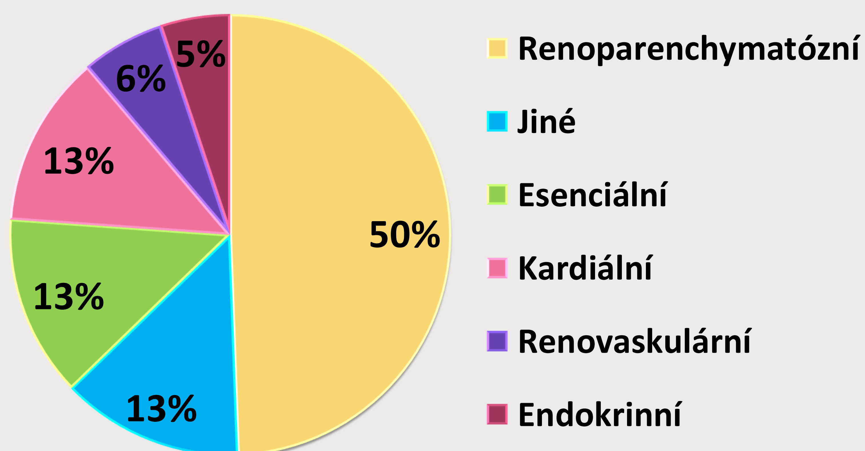
Graf č. 1 – Příčiny hypertenze u dětí indikovaných k léčbě antihypertenzivy
